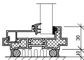
Profil ved gulv
