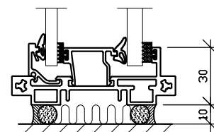
Profil ved gulv - dobbeltglas
