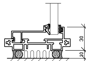
Profil ved gulv - enkelt glas
