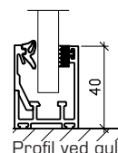
Profil ved gulv
