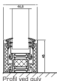
Profil ved gulv
