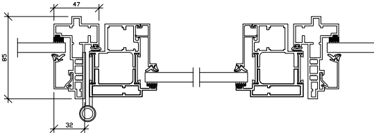
Vandret snit: Samling vægprofil med helglasdør/glasrammedør
