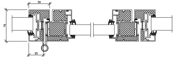
Vandret snit: Samling vægprofil med glasrammedør
