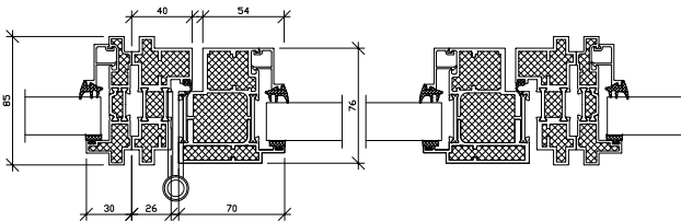
Vandret snit: Samling vægprofil med glasrammedør
