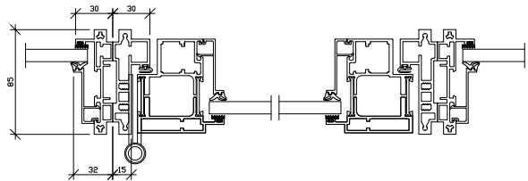
Vandret snit: Samling vægprofil med glasrammedør
