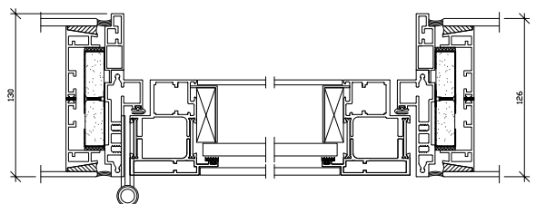
Vandret snit: Samling vægprofil med glasrammedør
