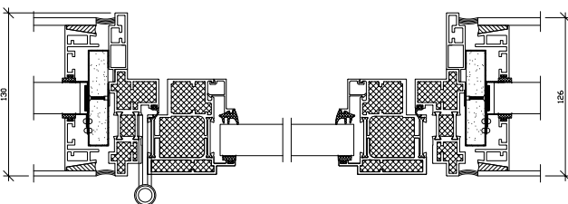
Vandret snit: Samling vægprofil med glasrammedør
