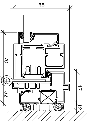
2. Samling glas/glasdør
