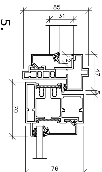
Samling glas/glasrammedør
