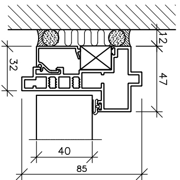
Samling glasrammedør/væg
