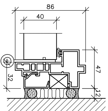
Samling glasrammedør/væg, hængsel
