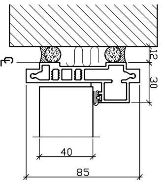
Samling Trædør/væg
