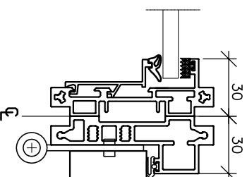
Samling trædør/element hængsel
