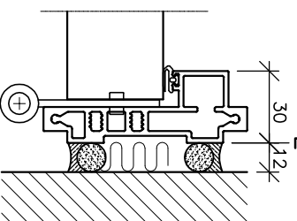
Samling Trædør/væg, hængsel
