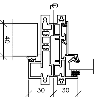
Samling trædør/element
