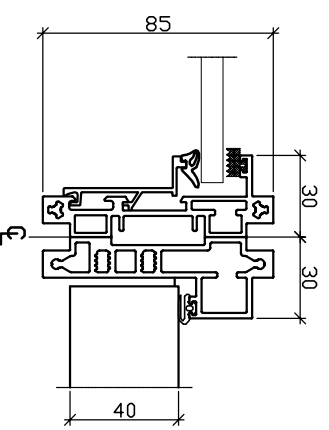
Samling trædør/element
