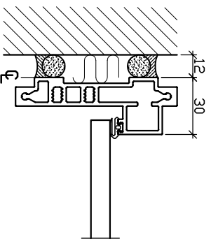
Samling Helglasdør/væg
