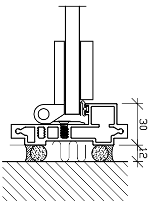
Samling helglasdør/væg, hængsel
