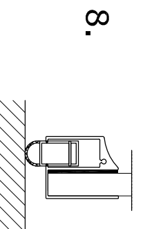
Tilslutning ved gulv med bundtrækning
