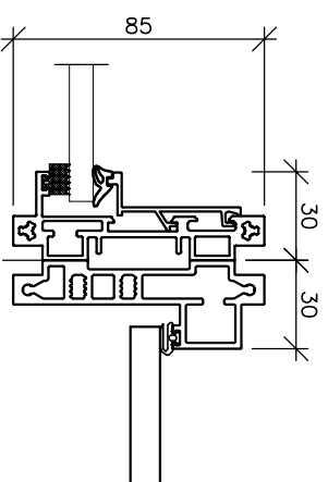
Samling helglasdør/element
