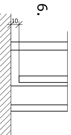
Tilslutning ved gulv
